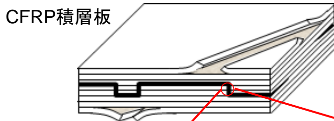
トランスバースクラック
