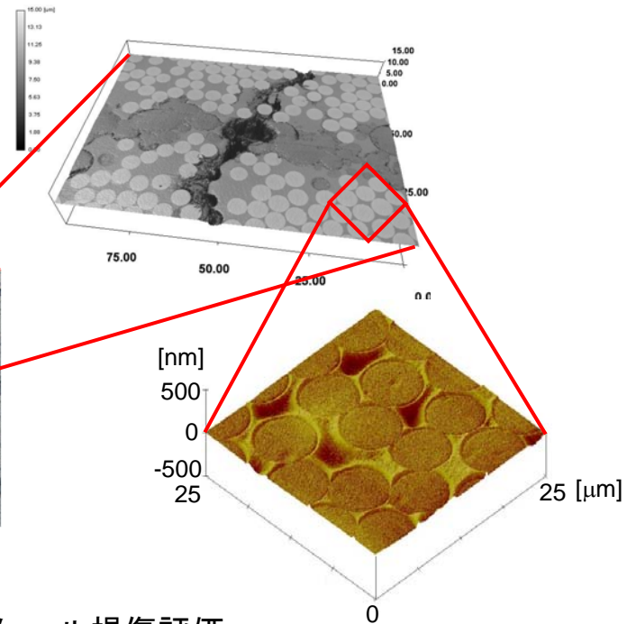
CFRPのマルチスケール損傷評価
