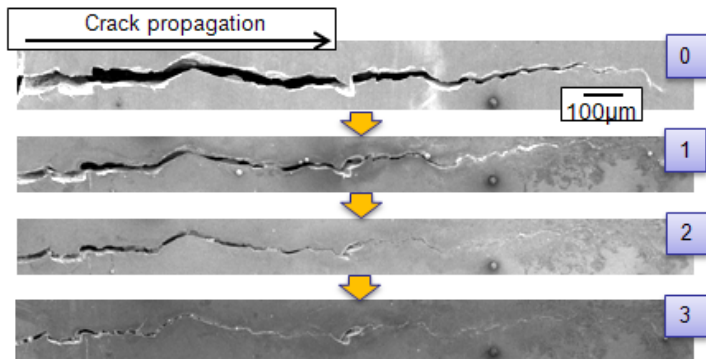
高密度電子衝突による金属疲労き裂の治癒
