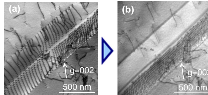
(a) 電子衝突前
